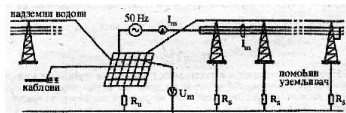
Slika 3: Merenje impedance uzemljenja, napona dodira i napona koraka
