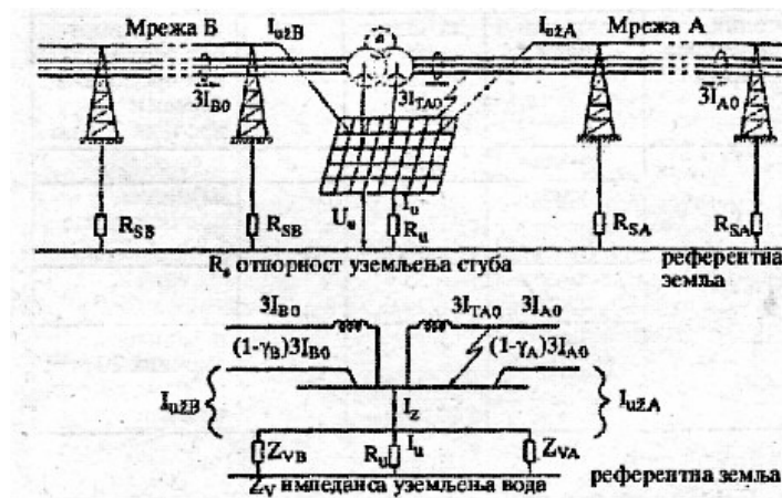
Slika 2: Raspodela struja u sistemu uzemljenja
